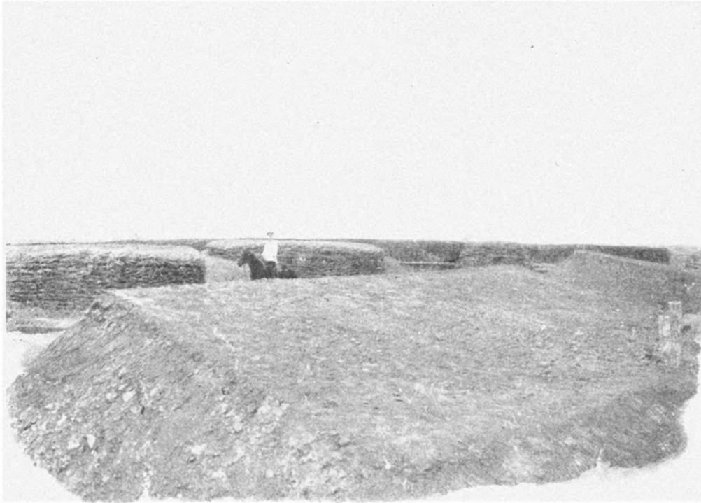
Фортъ „Лѣсной“ № 6 въ законченномъ видѣ при укрѣпленіи позиціи у дер. Чишанькоу.
