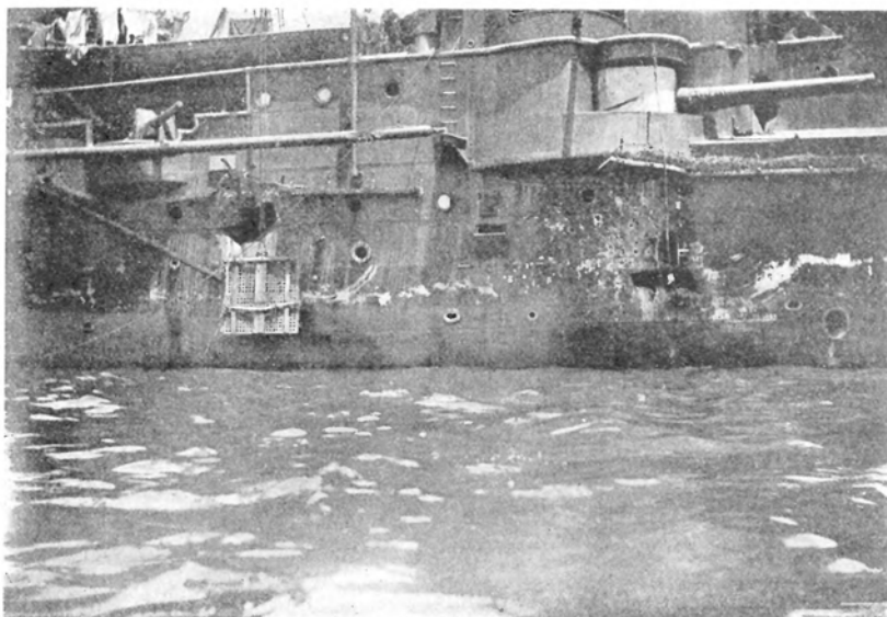
Пробоина у ватерлиніи на „Олеѣ“.
