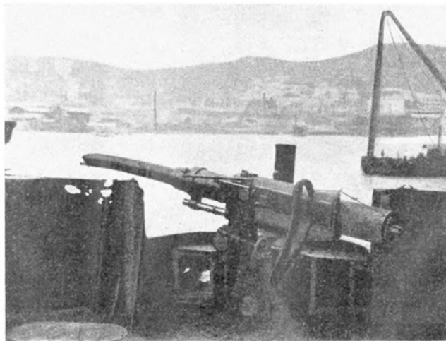
75 мм. пушка послѣ попавшаго въ дуло снаряда.
