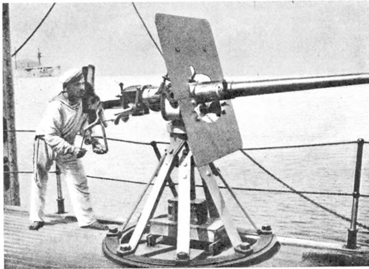
47 мм. пушка Гочкеса.
