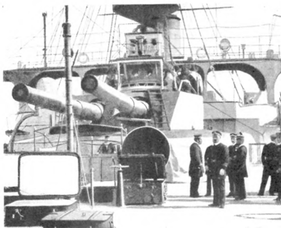
12-дюймовыя орудія на броненосцѣ.
