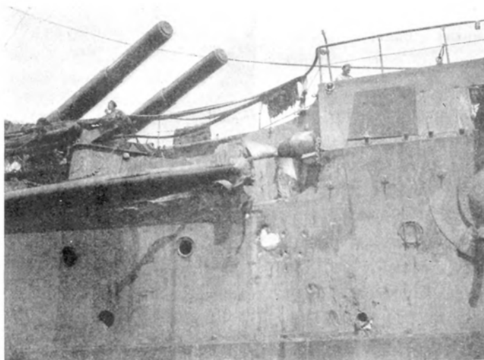
Пробоина отъ 8" м. японскаго снаряда на „Цесаревичѣ“.
